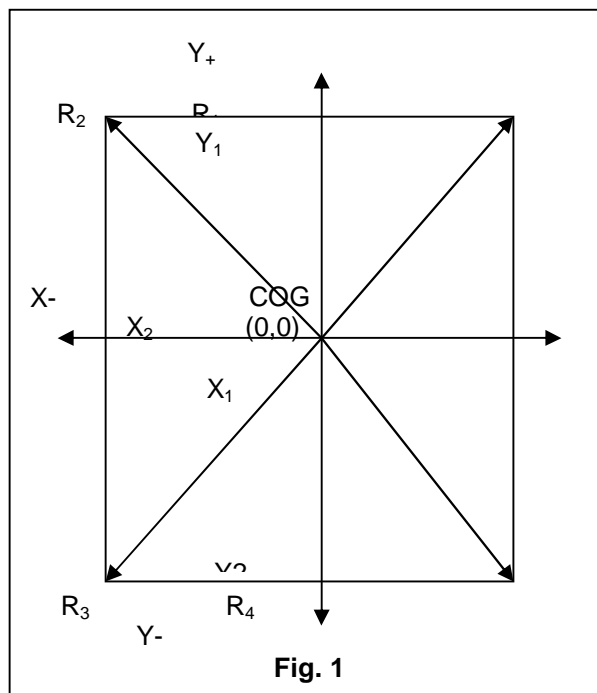
Fig. 1 Pattern Statistical Parameters
